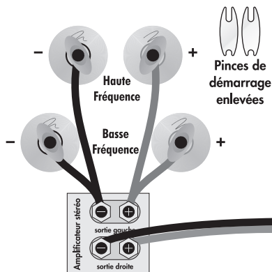
Fig. 2: Raccord à deux fils. Un canal illustré.
