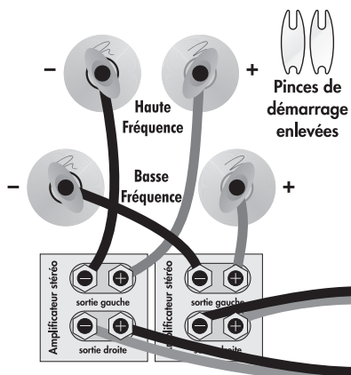
Fig. 3: Raccordement par bi-amplification horizontale. Un canal illustré.
