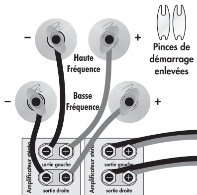
Fig. 4: Raccordement par bi-amplification verticale. Un canal illustré.
