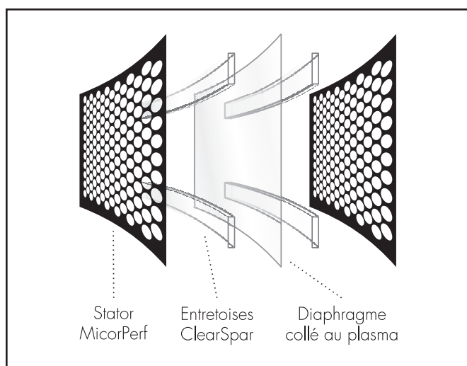
Figure 12. Vue en coupe d'un transducteur électrostatique XStat. Remarquez la simplicité due au petit nombre de pièces utilisées.
