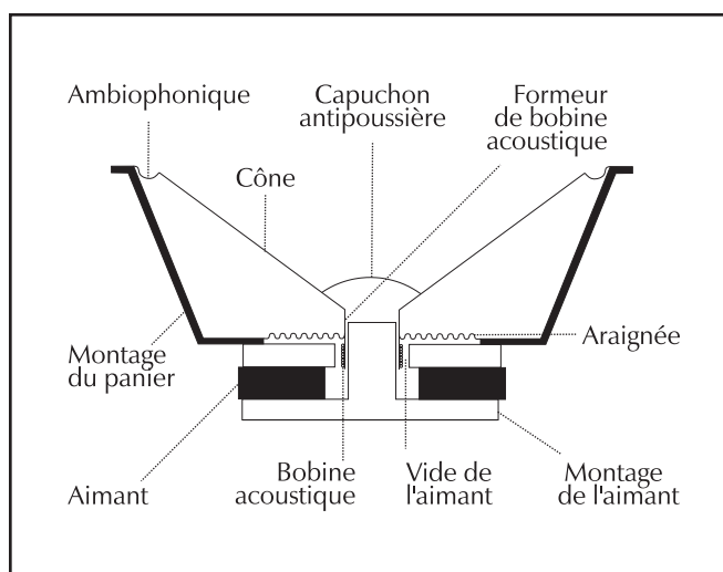
Figure 13. Vue en coupe d'un haut-parleur à bobine en mouvement typique. Remarquez la complexité due au grand nombre de pièces utilisées.
