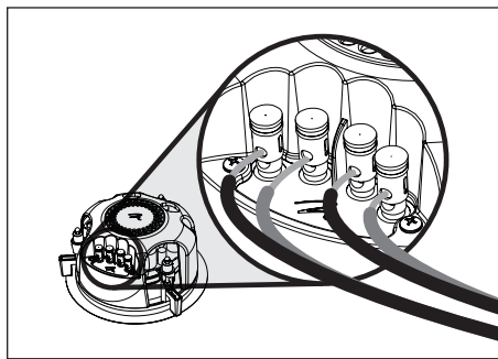
Figure 2. Raccordement du Helos 22 pour une utilisation en stéréo.
